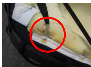
9、側面部のバンドのS字フックは画像のようにシートの金属部に引っ掛け固定します。
