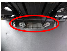
19、助手席にテーブルが付いている際は、6箇所のネジをプラスドライバーを使い取り外しておきます。
